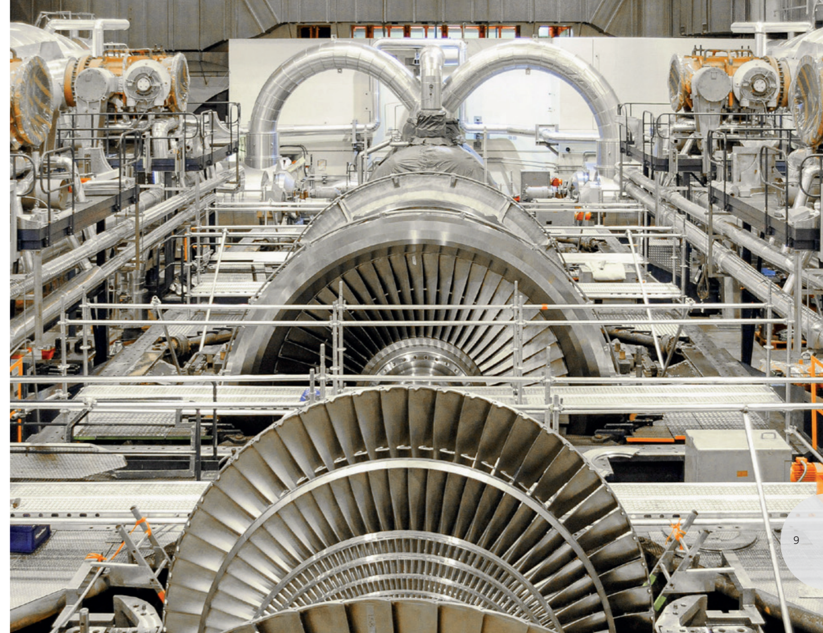
Niederdruckturbinen im Kernkraftwerk Leibstadt
